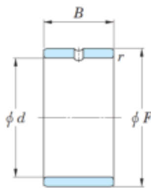
JR.JS1
