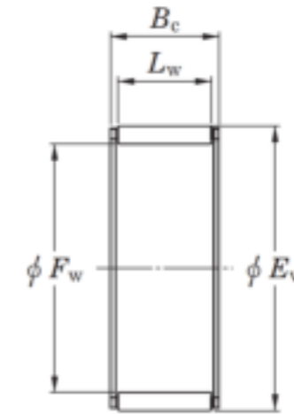
WJ, WJC
