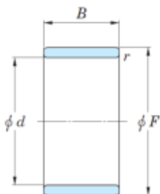
JR, IM..P
